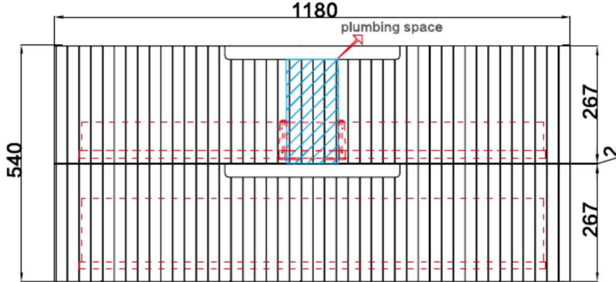
CAWH42-1200
