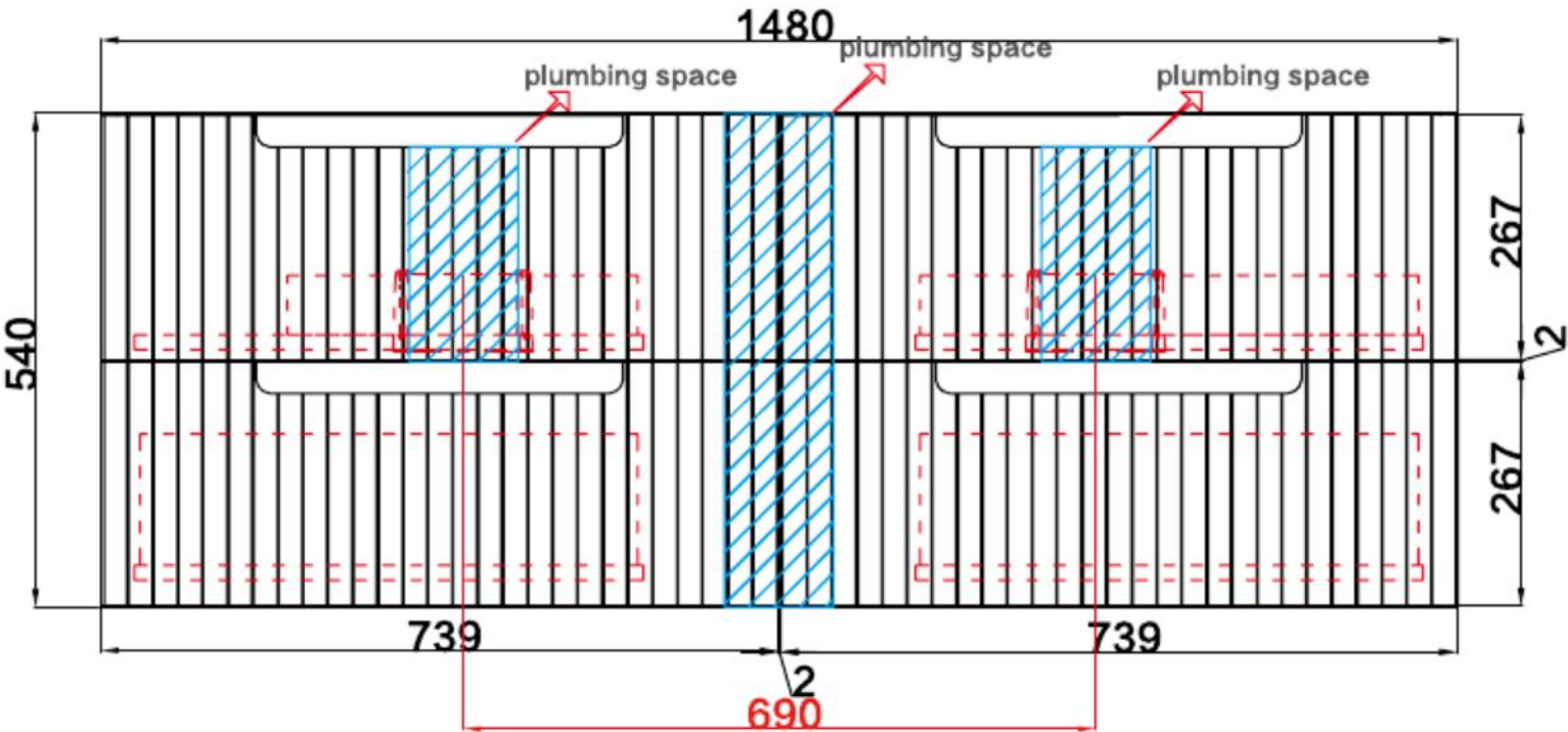
CAWH42-1500
